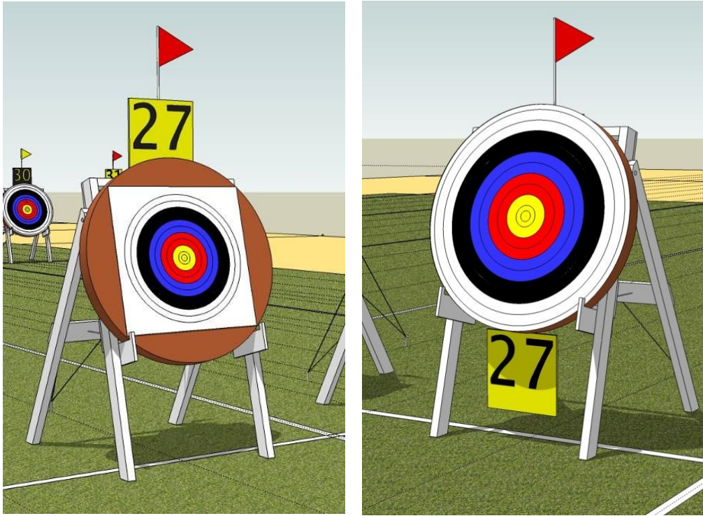
Figura 11. Configuraciones aceptables de parapetos – Vista frontal
