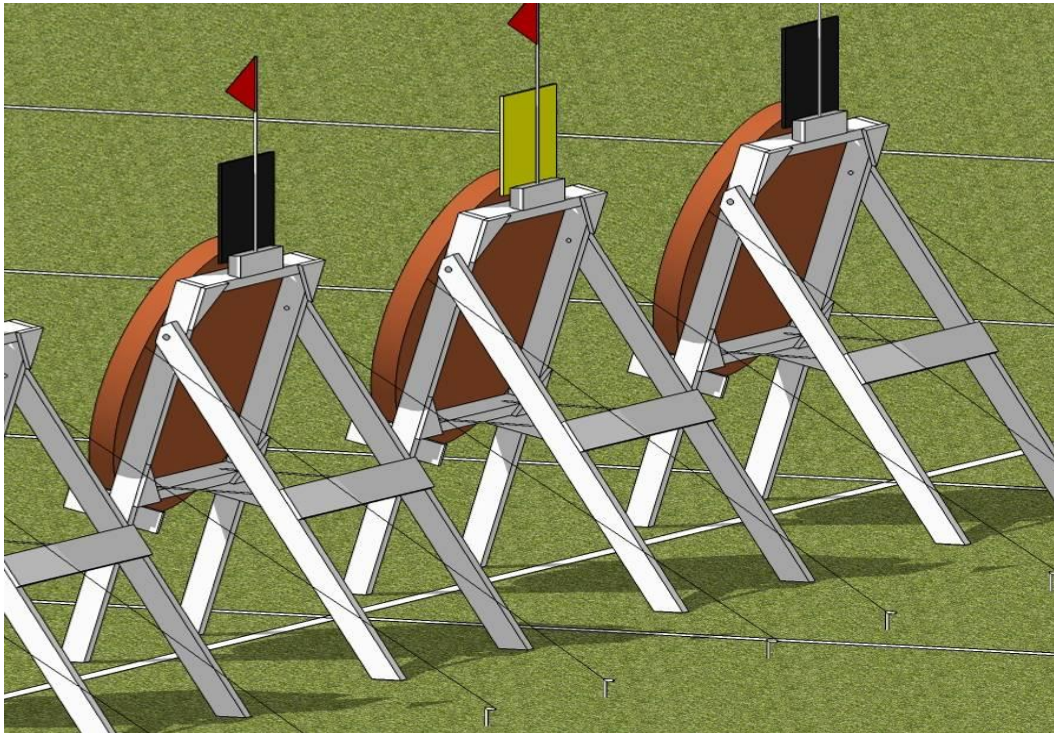
Figura 12. Vista posterior de los parapetos donde se aprecia su fijación
